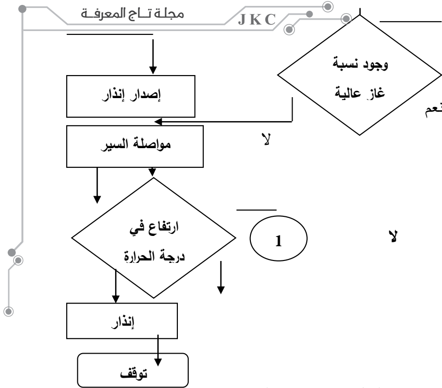
الشكل (2-6) يوضح فيه المخطط الانسيابي للروبوت
