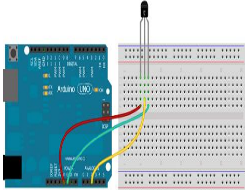
الشكل (20-5) يوضح طريقة توصيل حساس الحرارة بلوحة المتحكم أروينو .
