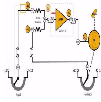
طريقة عمل المحرك
