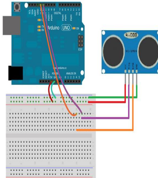
الشكل (21-5) يوضح توصيل حساس الموجات ما فوق الصوتية بلوحة المتحكم أروينو .
