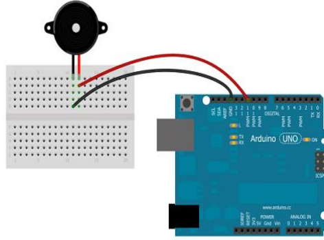
الشكل (5-18) يوضح توصيل الطنان الكهربائي بلوحة المتحكم أروينو .
