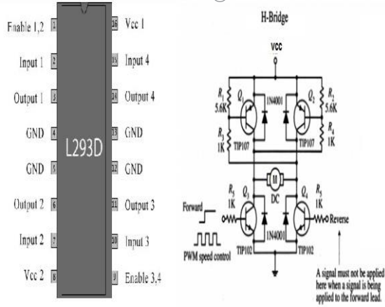
جزء من التركيب الداخلي لشريحة
