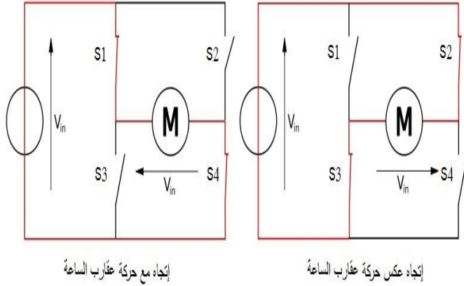
الشكل (4-5) يوضح اتجاه حركة المحرك .
