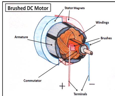
الشكل (3-5) يوضح تركيب محرك التيار المستمر .
