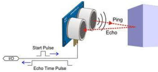
الشكل (13-5) يوضح طريقة عمل حساس ما فوق الصوتية .
